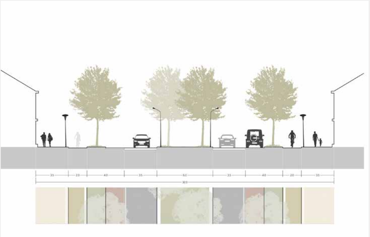
Beoogd profiel Borgharenlaan
